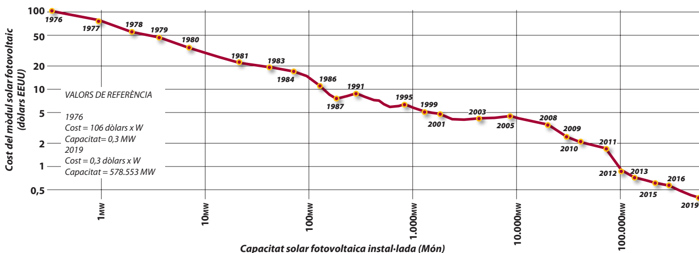
Figura 5. El cost minvant de la tecnologia solar: un 99.6% menys des de 1976
