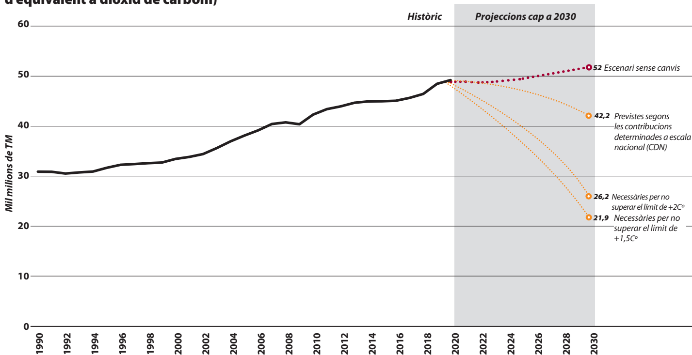
Figura 8. Emissions de gasos d'efecte hivernacle: històric i escenaris (milers de milions de tones mètriques d'equivalent a diòxid de carboni)
